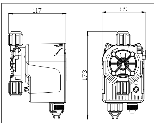
Рис.8 Габаритные размеры
